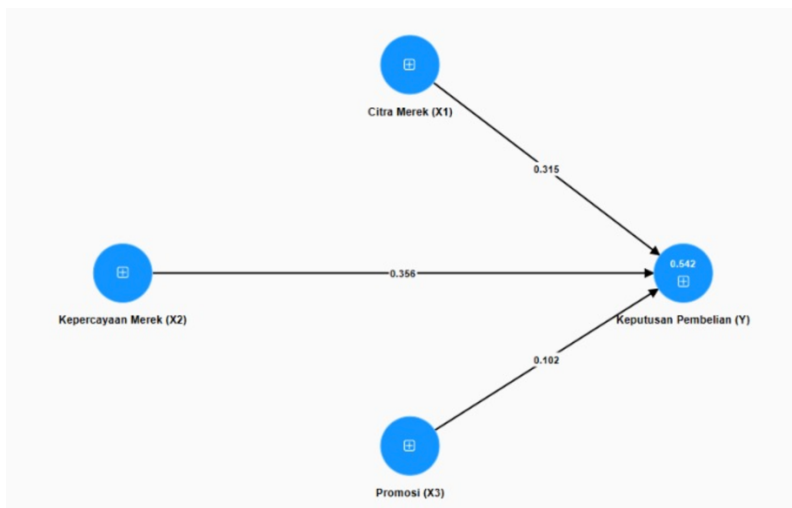
Lampiran 5. Hasil Inner Model pada SmartPLS 4.0
