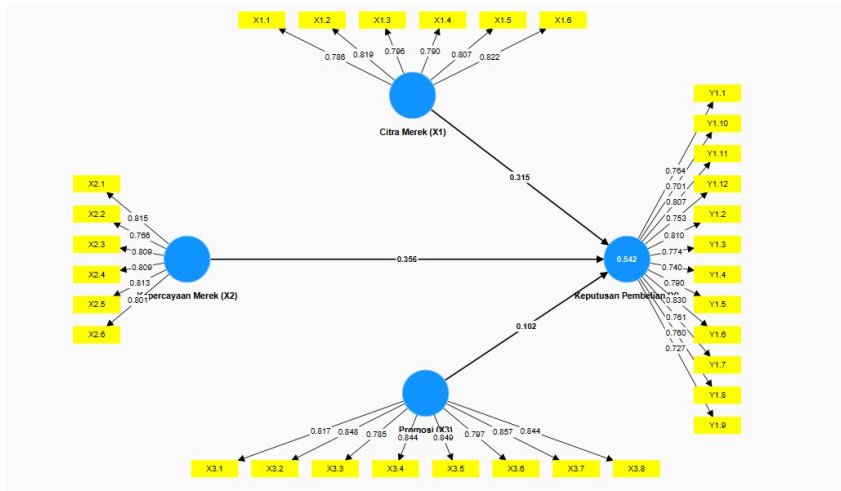
Lampiran 4. Hasil Outer Model pada SmartPLS 4.0
