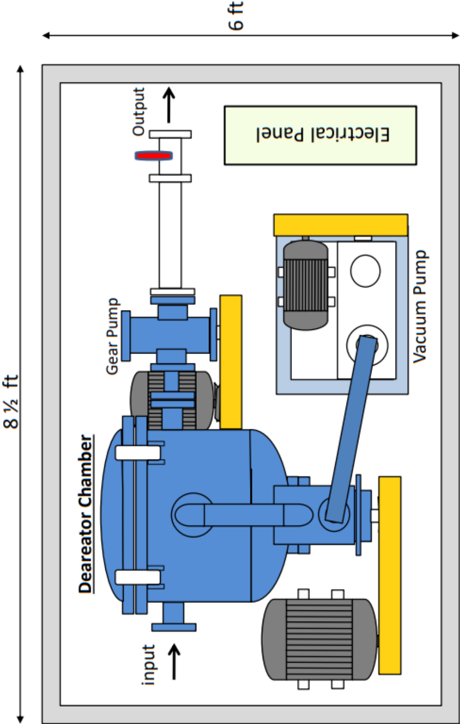
Lampiran 4 Gambar Dimensi Plat Mesin dan Denah Mesin Deaerator Digrease Plant
